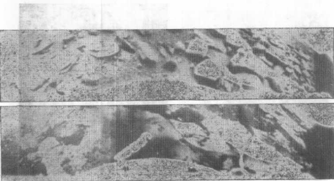
苏联“金星9”号和“金星10”号拍摄的金星表面两个不同地方的周围景象。在两张照片里，地平线都在右上方。注意表面岩石被侵蚀的状态。
