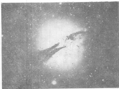
半人马座 A (NGC 5218)。大概是碰撞中的一个巨椭圆星系和一个漩涡星系。我们在后面看到的是后者被毁坏的旋臂。它距我们 1400 万光年远，它的射电波瓣长达 300 万光年。
