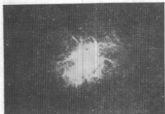
金牛座的蟹状星云。距离为6000光年，该星云是人类观察到的1054年的超新星爆炸的残留物质形成的。星云的纤状部分以每秒1100公里的速度向外扩散。尽管它已经扩散了差不多1000年，但它每秒钟向空中发射的能量仍比太阳高大约10万倍。星云中心是一颗不断搏动的高密度中子星，搏动频率约为每秒30次。
