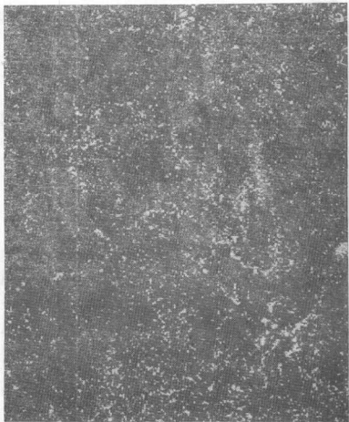
大型宇宙结构图。百万个最明亮的星系图样。所有的星系都在离地球10亿光年的距离以内，每一个小方块都是一个含有几十亿颗恒星的星系。本图是根据望远镜的观察结果绘制的，是加利福尼亚大学立克天文台的唐纳德·沙恩和卡尔·伏世图花了12年的时间完成的。
