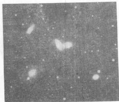
史蒂芬五重奏，1877 年发现的一群五个显然相互作用的星系。
