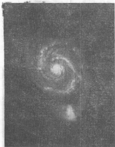
漩涡银河系M51 [梅西耶星云星团表中第51号天体，也称为NGC 5194]。1845年罗斯爵士发现了这个“星云”的漩涡结构。这是观察到的有这种结构的第一个星系，距地球1300万光年。
