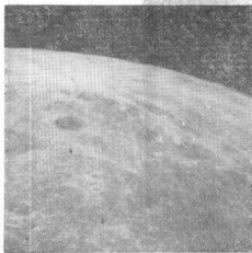
月球上有辐枪射纹的布鲁诺环形山(顶部)。
