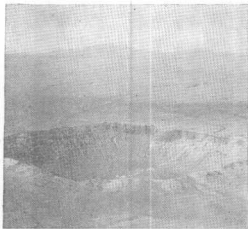
亚利桑那的陨星坑，宽1.2公里，大概是15000年至4万年前由一个直径25米的铁块以每秒15公里的速度撞击地球形成的。撞击所释放出来的能量相当于400万吨级核爆炸所释放出来的能量。
