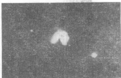
大约有5000万光年远的碰撞星系，碰撞前后经历了一亿多年。
