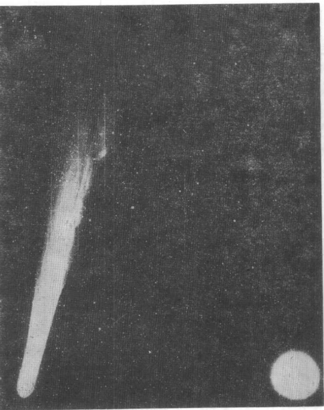
一张1910年拍摄的哈雷彗星和金星
