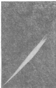
雅谷一英彗星，是两个热心的日本业余天文学家在1965年发现的，这个彗星的尾巴大约有5000万公里长。（迈克尔·贝尔顿摄于美国基特峰国家天文台）
