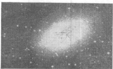
NGC 147 是伴随M 31 的小椭圆星系。它大概包含10亿个太阳。从那些恒星的一些行星上观看，可看到一个辉煌灿烂的M31 图象。
