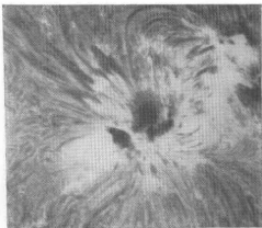
一组太阳黑子在氢红光下的近镜头。太阳黑子区的温度相对较低，但磁场很强。相邻的黑色“针状”区止是在它的强磁场下取向的。临近的明亮的“海滨”与太阳风出现有关。
