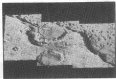
火星卡普里·查斯马北面斜坡上的一个环形山。由于凹陷处逐步在扩大，这个环形山已经开始断裂，并且出现侵蚀现象。（“水手9”号拍摄的拼合照片）
