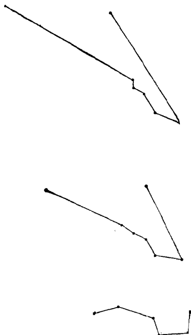
上图：100 万年前的北斗七星
