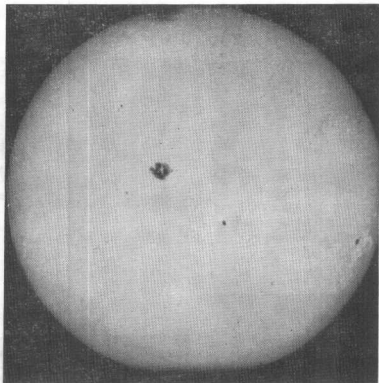
太阳光球——太阳四周的地球域，普通的可见光就从这里向太空辐射。 此图是在接近最大太阳黑子活动时拍摄的。
