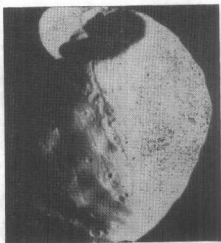
火卫一，火星最内侧的卫星。斯蒂克尼环形山在它的顶端。假如形成这个环形山的撞击物体稍大一点，火卫一就可能已经崩毁了（“海盜1”号轨道飞行器拍摄的照片）。
