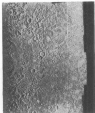
在灼热的水星表面的卡洛里斯大盆地的边缘地带（图中左边看到的同一中心的裂缝和山脊）。“水手10”号拍摄的拼合照片）。
