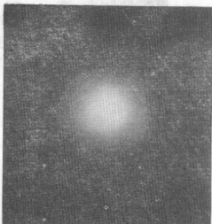
已知的最巨大的星系M87。它是靠近室女座巨大星系团中心，距离大约为4000万光年远的一个巨型椭圆星系。
