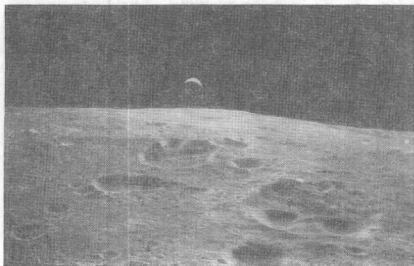
地球从月球上起伏的小山和错综垂迭的环形山升起。（“阿波罗”号轨道飞行器拍摄的照片）
