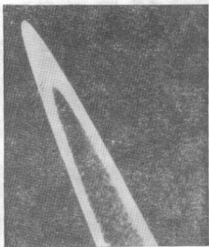
木星的部分光环图。“旅行者1”号发现，“旅行者2”号拍摄。木星在图外右下方。光环是由粒子组成的，似乎一直延伸到木星云端，可能处于不断产生和消失的状态之间；生于木星一所失散的物质，失于木星的云层之中。它比土星的光环要小得多，朦胧得多。因此，在“旅行者”号飞船之前，人们从未发现过这个光环。
