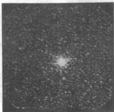
星空的x射线照片，显示出大天鹅x-1明亮光源（中心）。它大概是一个黑洞。由2号高能天体物理天文台在地球轨道上拍摄。
