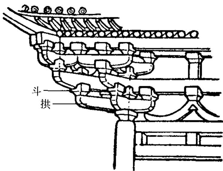
斗 拱
