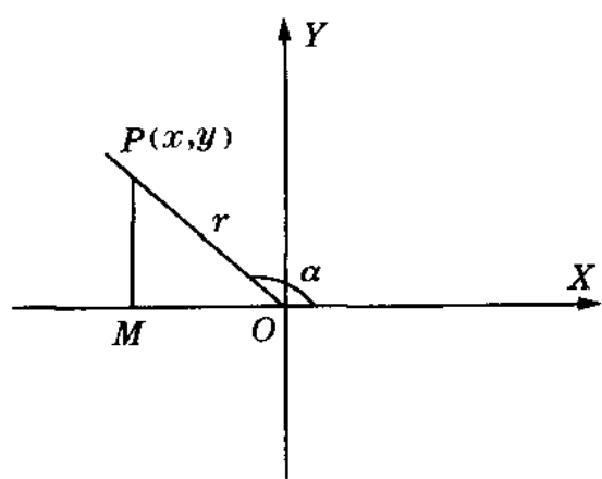
三角函数(二)
