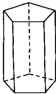
棱柱
