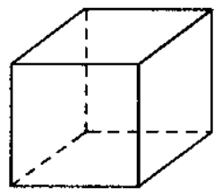
多面体
