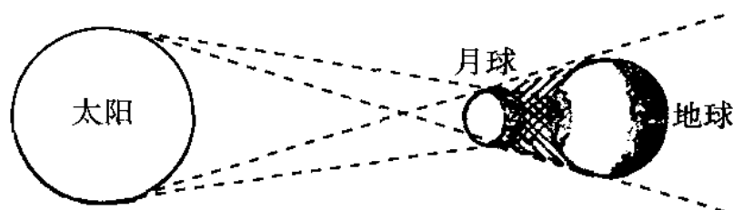
日 食
