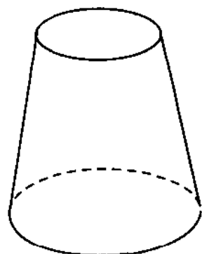
圆台
