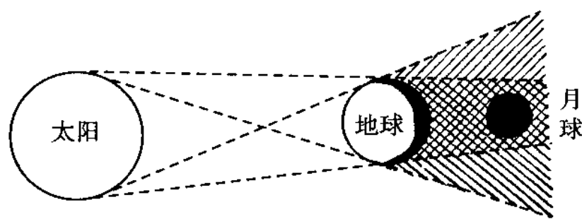
月食
