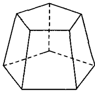
棱台
