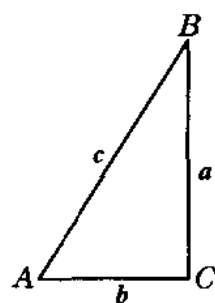
三角函数(一)
