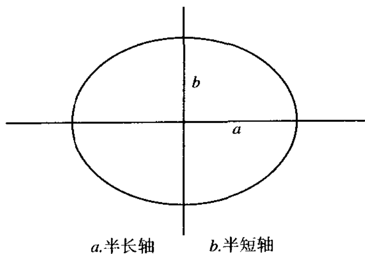
扁 率
