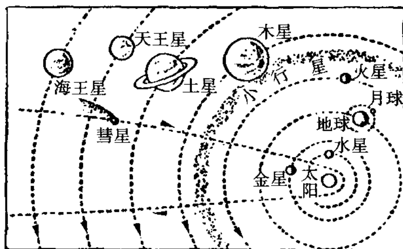
太阳系
