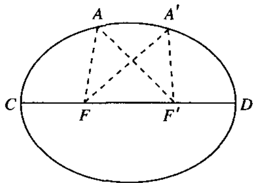
椭圆
