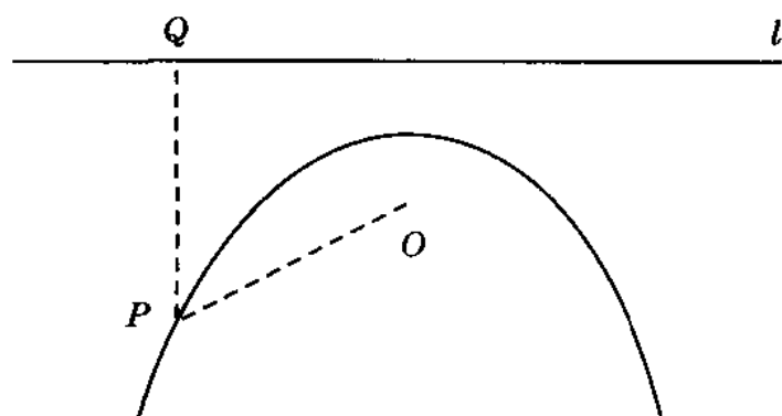
抛 物 线
