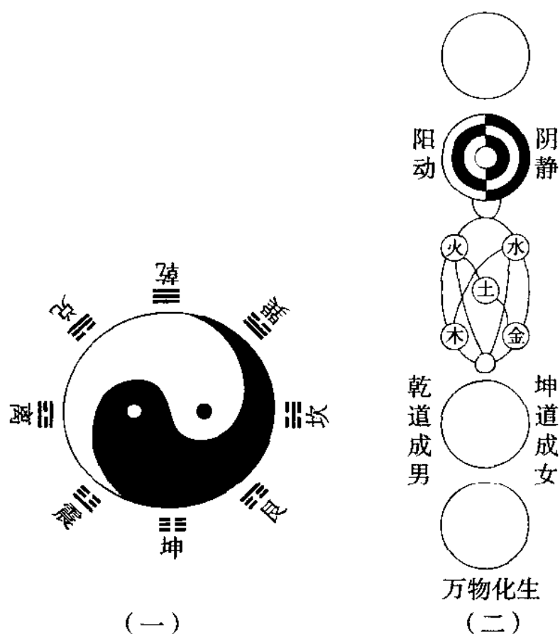
太极图
